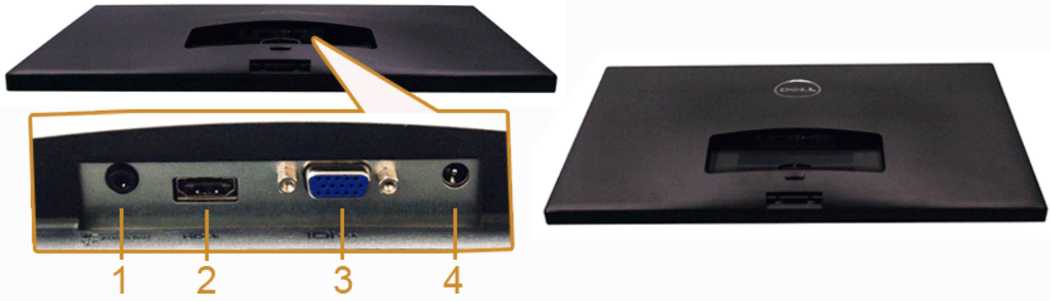
Ansicht von unten ohne Monitor-Standfuß
